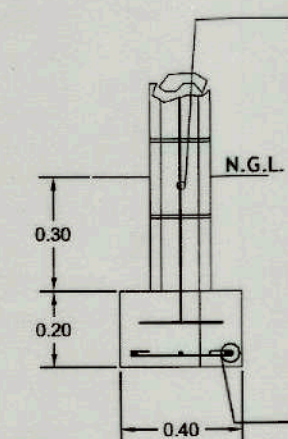
WALL FOOTING DET.
